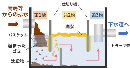
図1：グリストラップの構造
